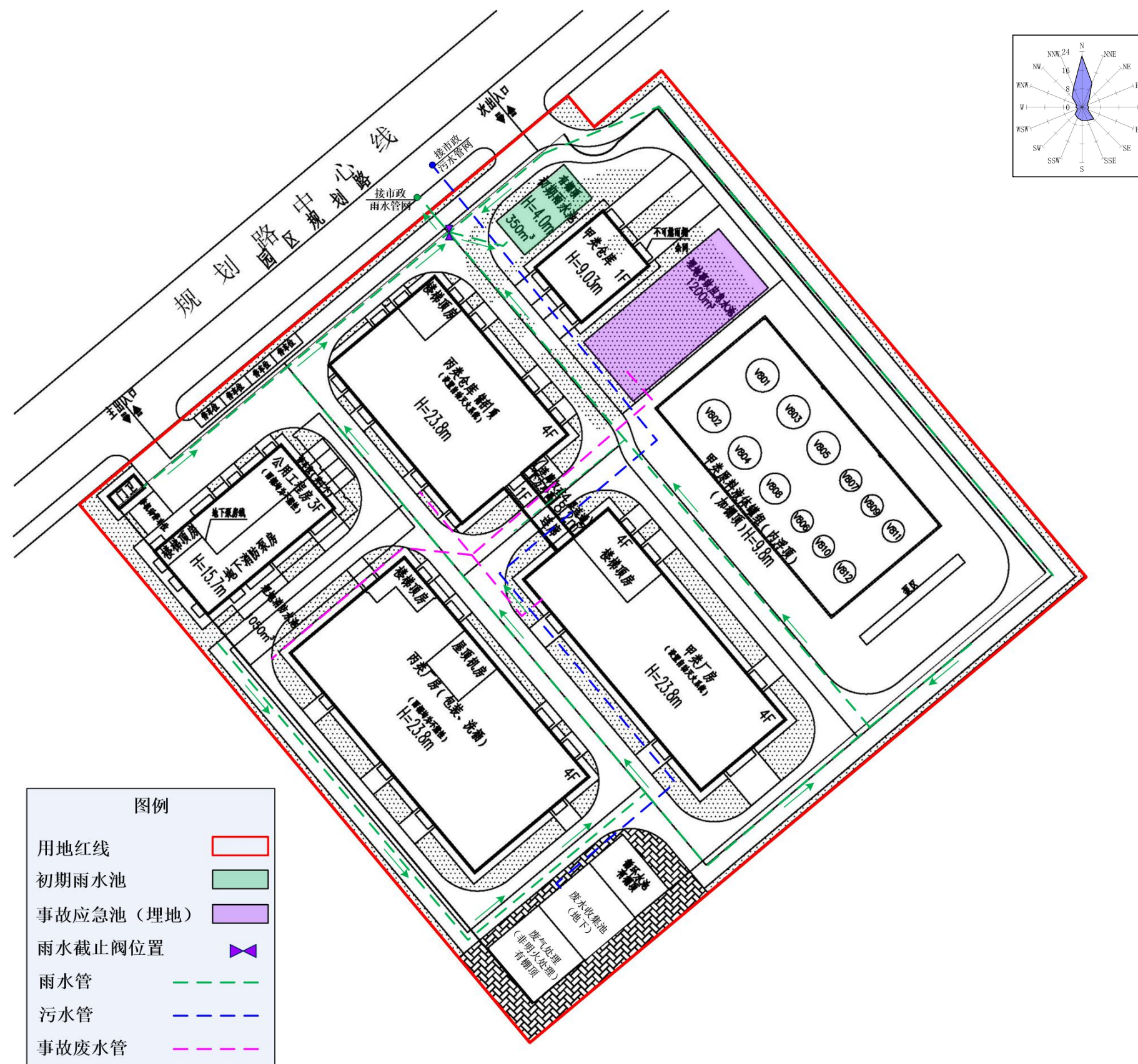
图 3.1-4 项目雨污管网图
