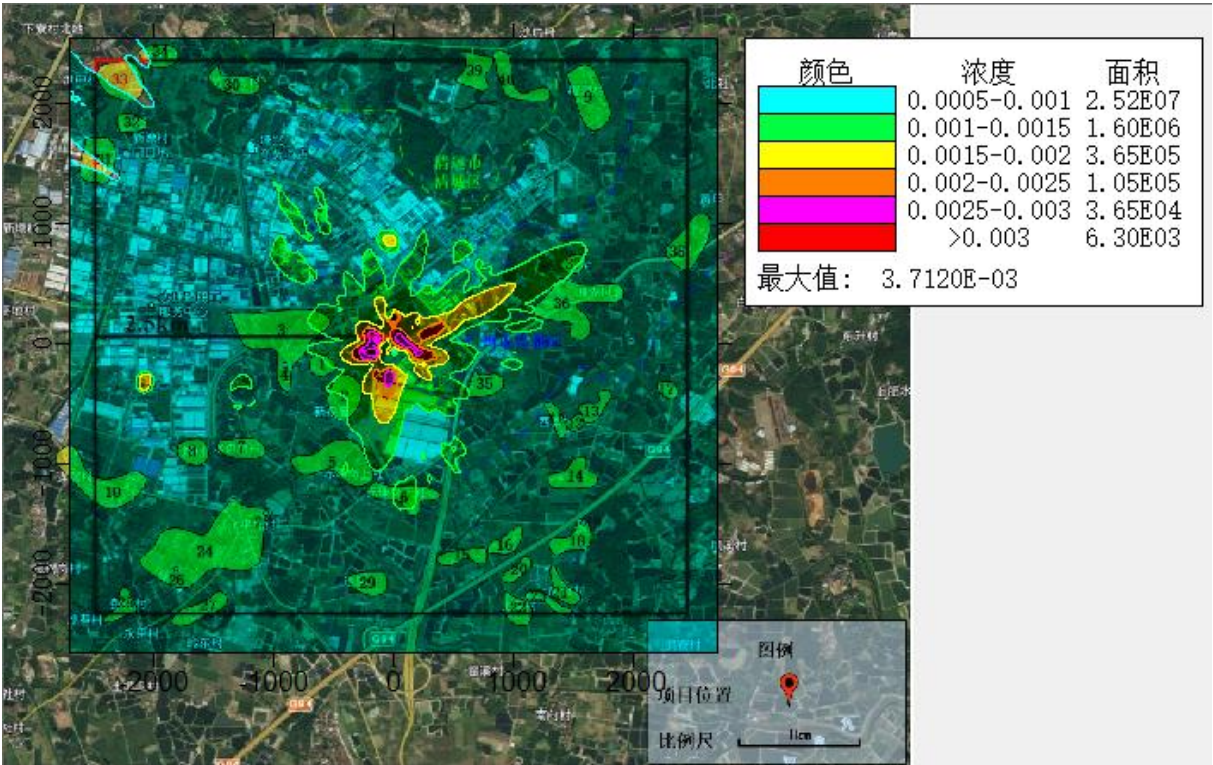
图 5.2-20 非正常排放时，苯乙烯 1 小时平均浓度贡献值等值线图
