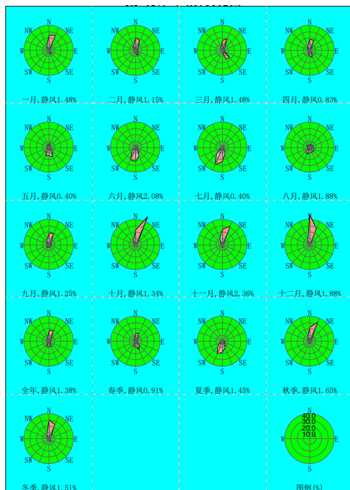
图 5.2-10 2020 年风频玫瑰图
