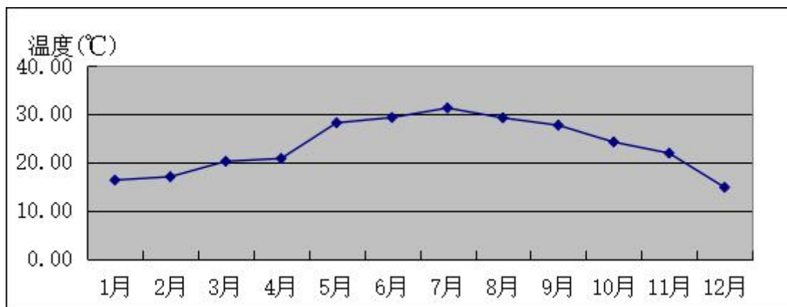
图 5.2-7 2020 年平均温度月变化曲线
