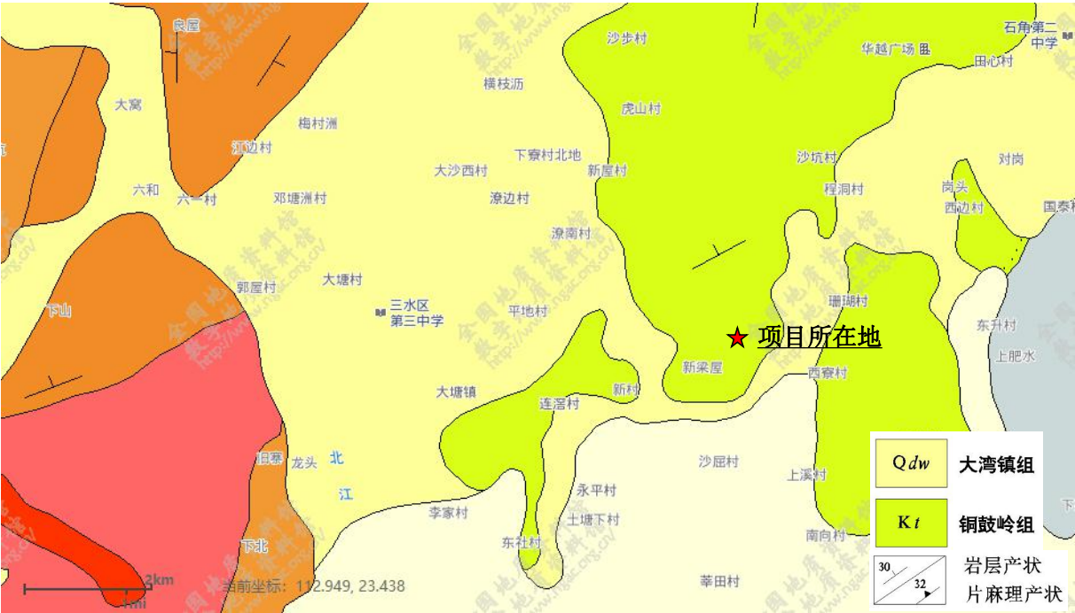
图 5.2-3 项目所在区域 1:20 万地质图
