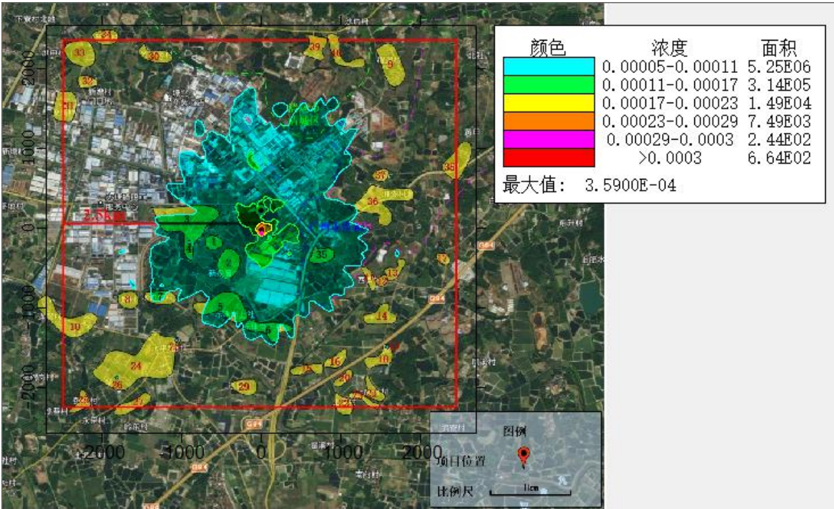
图 5.2-13 正常排放时，丙烯腈 1 小时平均浓度贡献值等值线图
