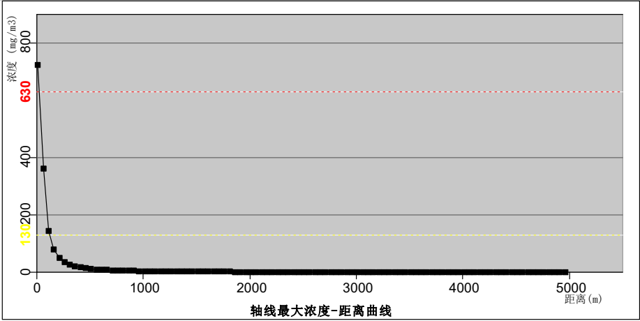
醋酸乙烯轴线最大浓度结果图
