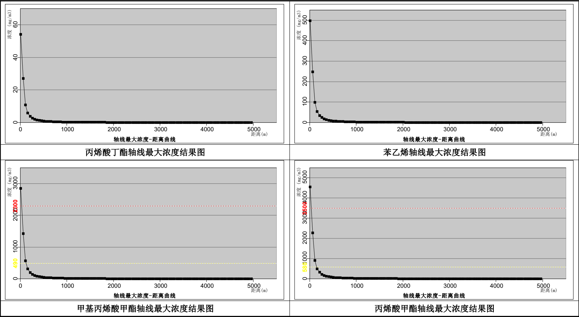
图 7.6-1 最不利气象条件下污染物轴线最大浓度结果图
