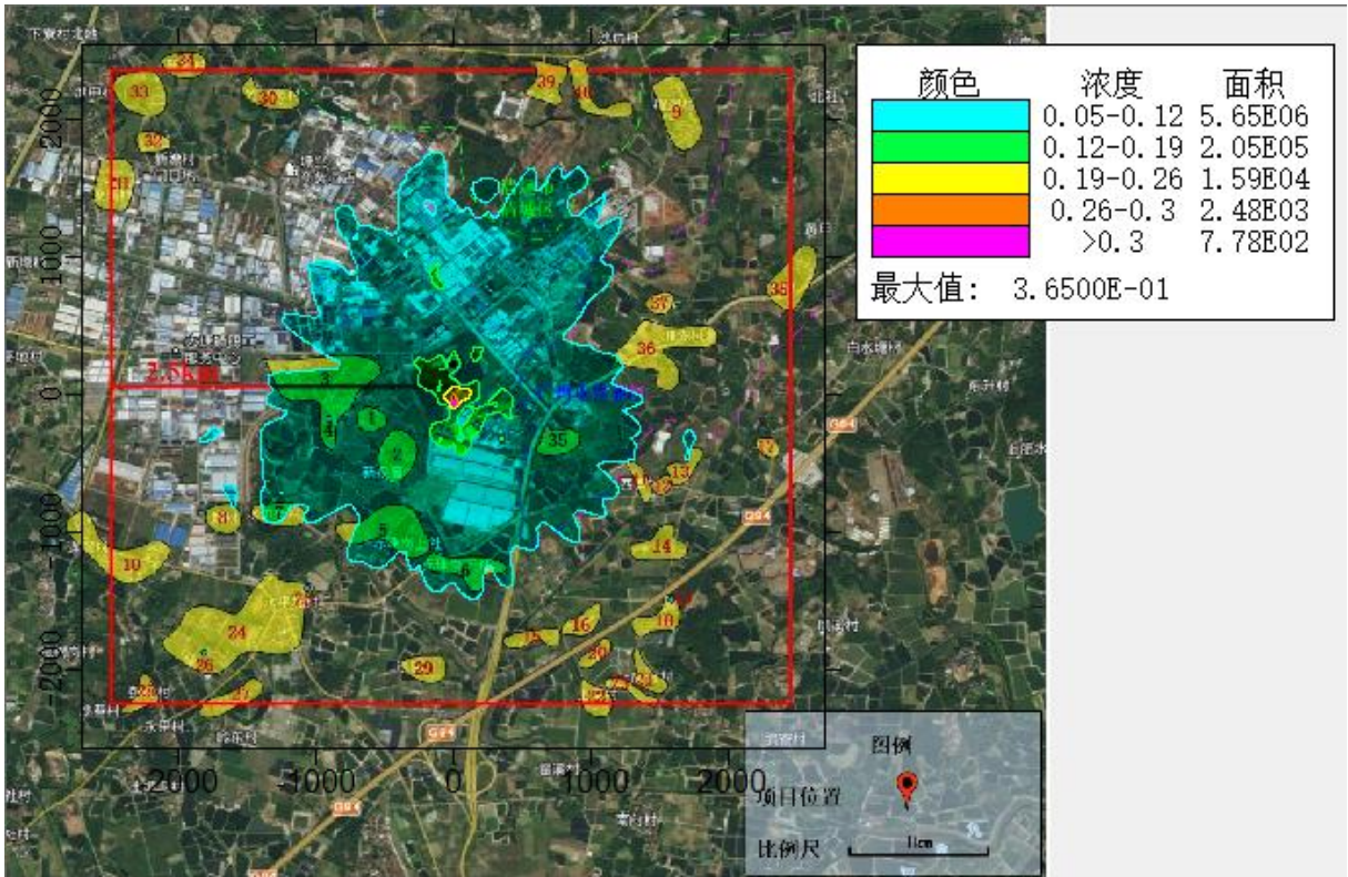
图 5.2-11 正常排放时，非甲烷总烃 1 小时平均浓度贡献值等值线图
