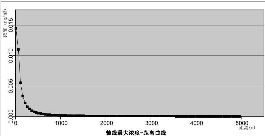
氢化 MDI 轴线最大浓度结果图
