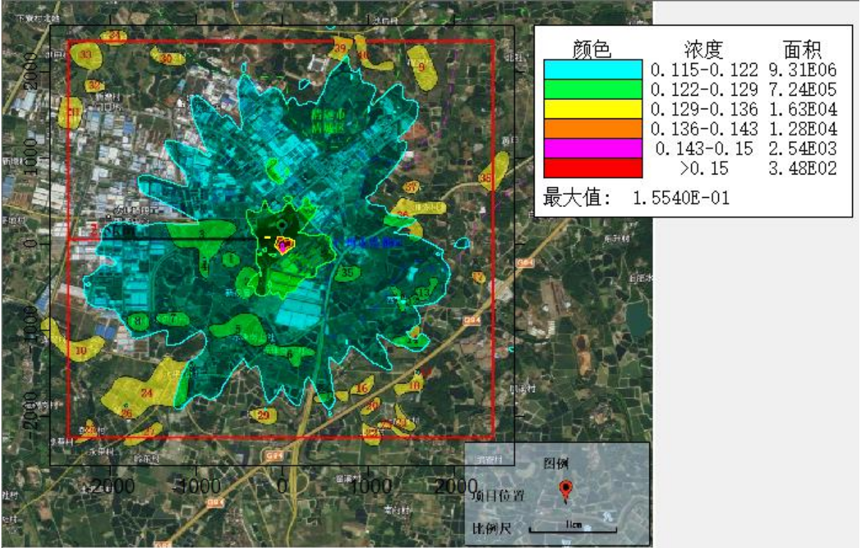
图 5.2-18 正常排放时，氨 1 小时平均浓度叠加值等值线图
