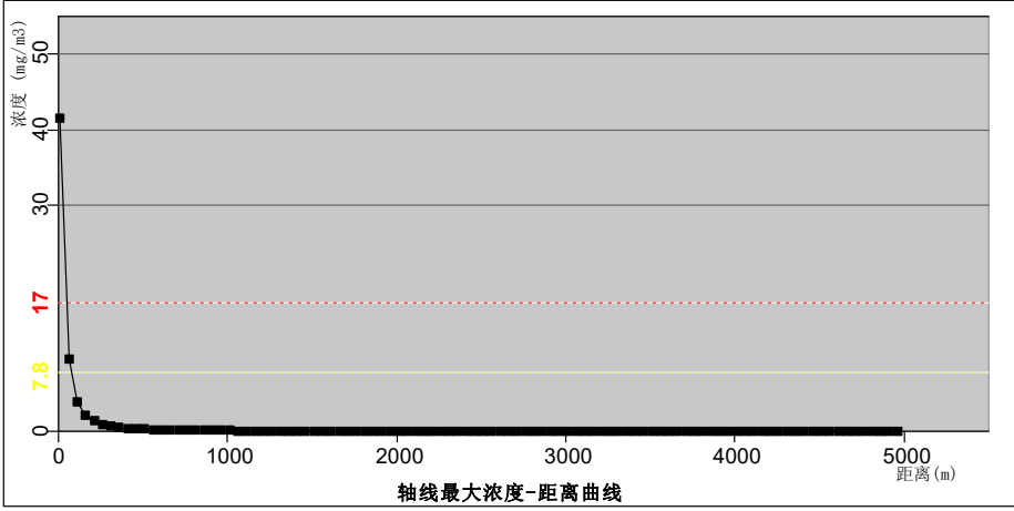
氰化氢轴线最大浓度结果图
