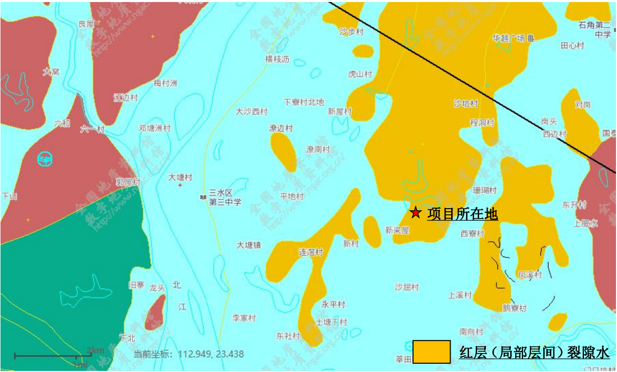
图 5.2-4 项目所在区域 1:20 万水文地质图
