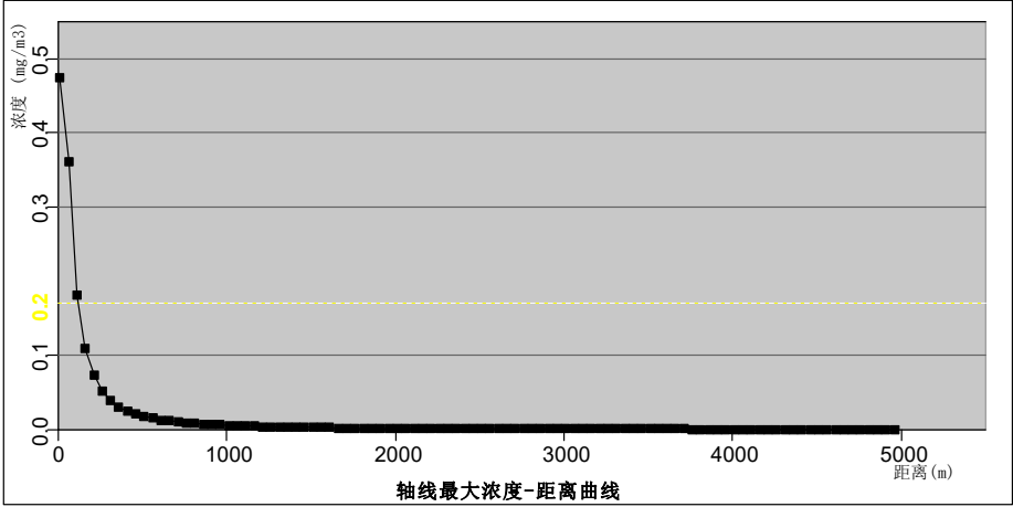
HDI 轴线最大浓度结果图
