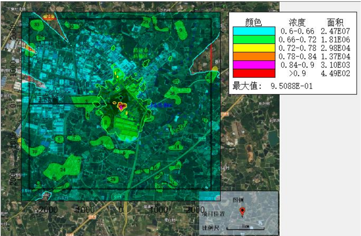
图 5.2-15 正常排放时，非甲烷总烃 1 小时平均浓度叠加值等值线图
