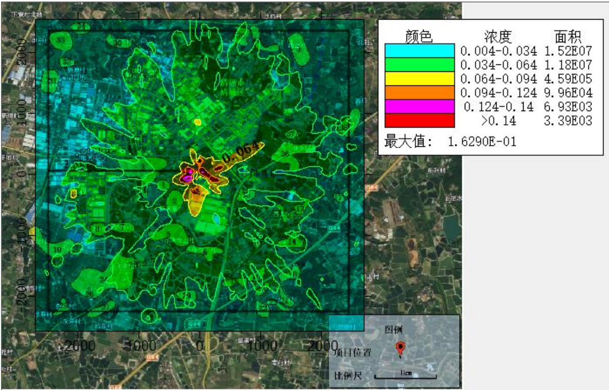
图 5.2-19 非正常排放时，非甲烷总烃 1 小时平均浓度贡献值等值线图
