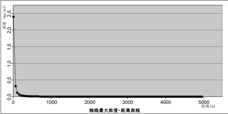
盐酸轴线最大浓度结果图
