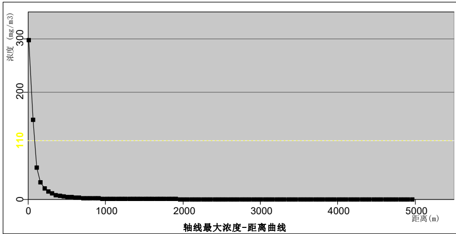
氨水轴线最大浓度结果图
