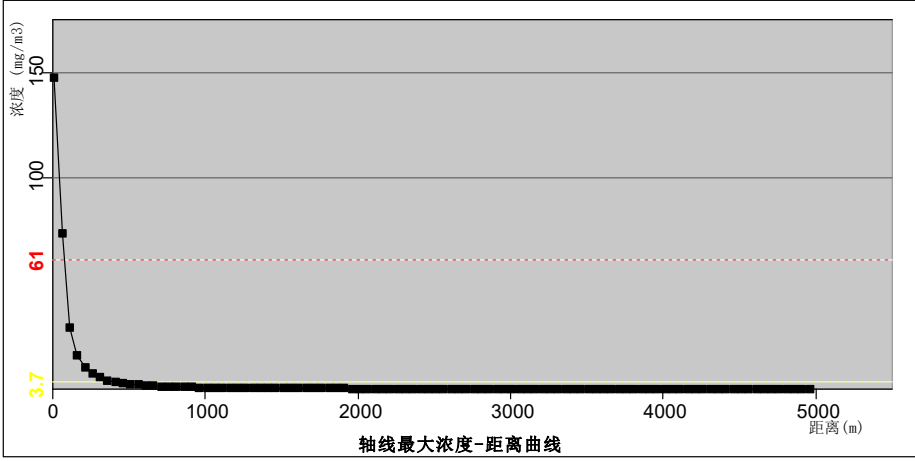
丙烯腈轴线最大浓度结果图
