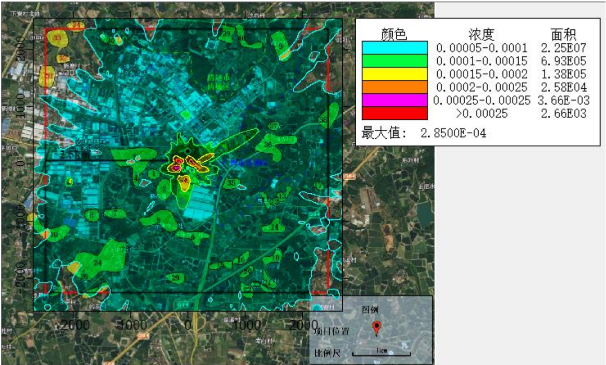
图 5.2-21 非正常排放时，丙烯腈 1 小时平均浓度贡献值等值线图
