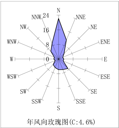
图 5.2-6 三水气象站风向玫瑰图（统计年限：2001-2020 年）
