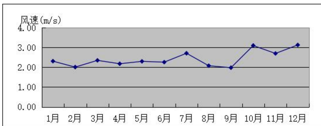
图 5.2-8 2020 年平均风速月变化曲线
