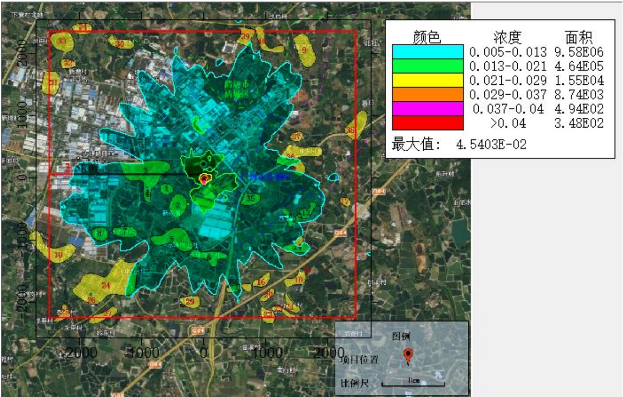
图 5.2-14 正常排放时，氨 1 小时平均浓度贡献值等值线图
