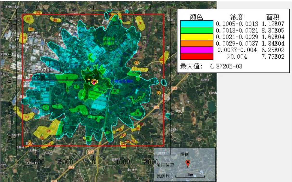
图 5.2-12 正常排放时，苯乙烯 1 小时平均浓度贡献值等值线图
