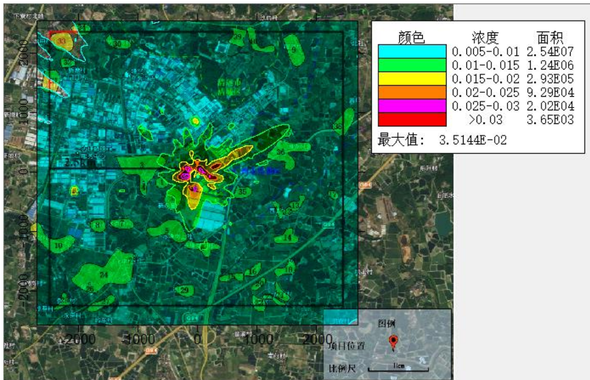
图 5.2-22 非正常排放时，氨 1 小时平均浓度贡献值等值线图
