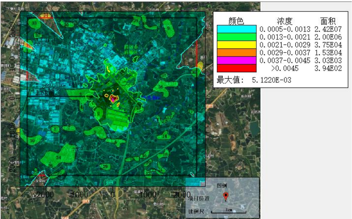
图 5.2-16 正常排放时，苯乙烯 1 小时平均浓度叠加值等值线图
