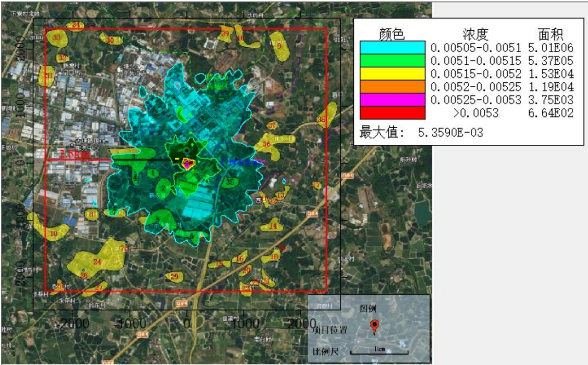
图 5.2-17 正常排放时，丙烯腈 1 小时平均浓度叠加值等值线图
