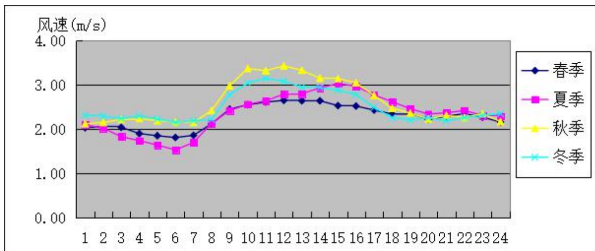
图 5.2-9 2020 年季小时平均风速日变化曲线
