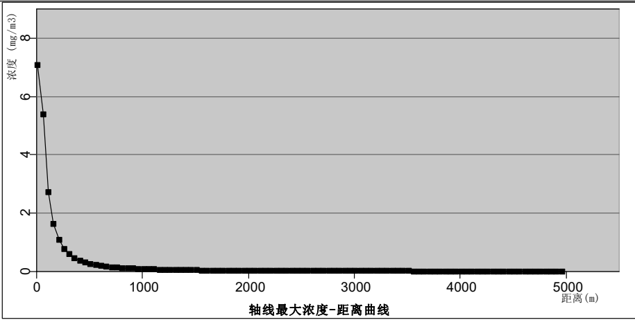
水合肼轴线最大浓度结果图
