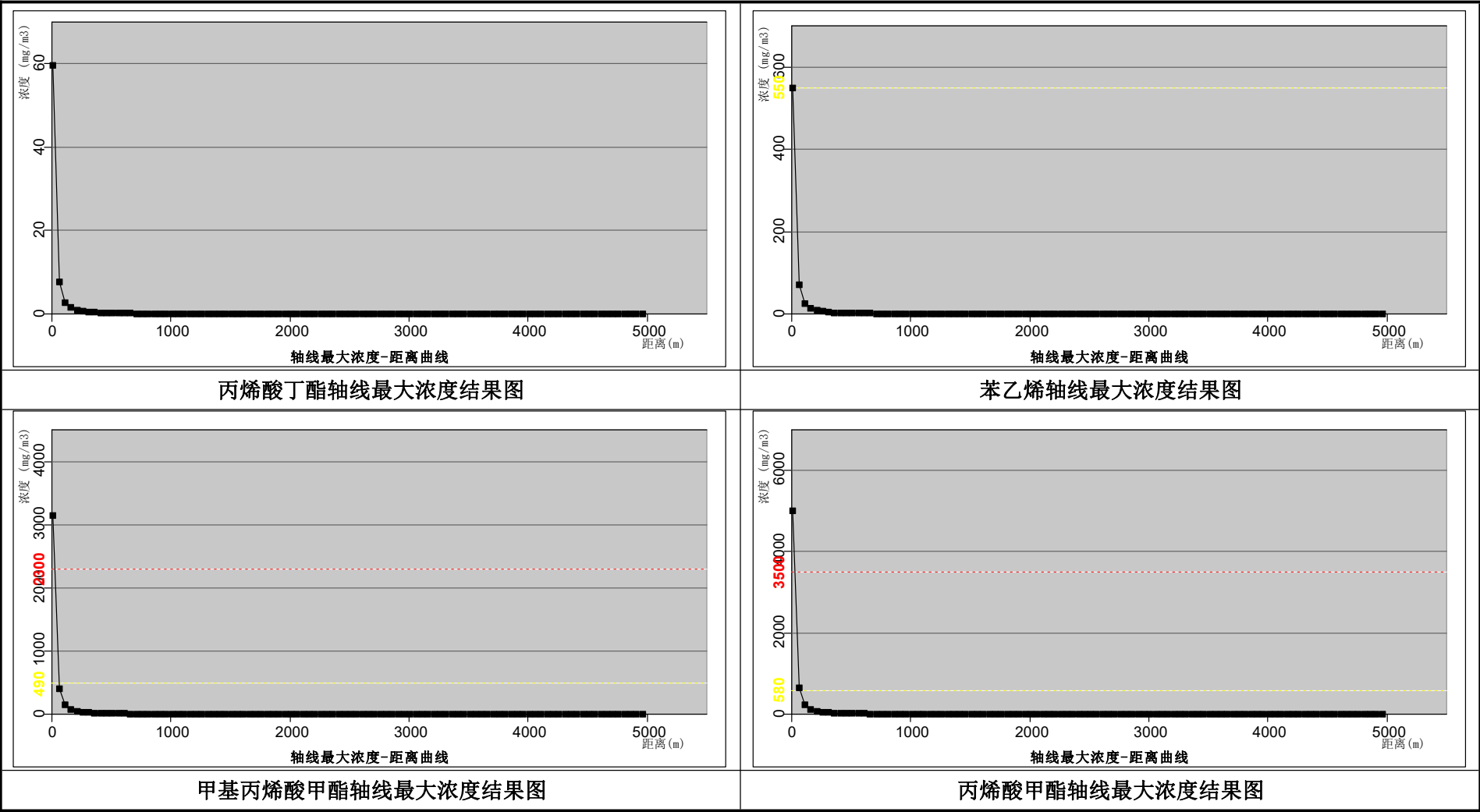
图 7.6-2 最常见气象条件下污染物轴线最大浓度结果图
