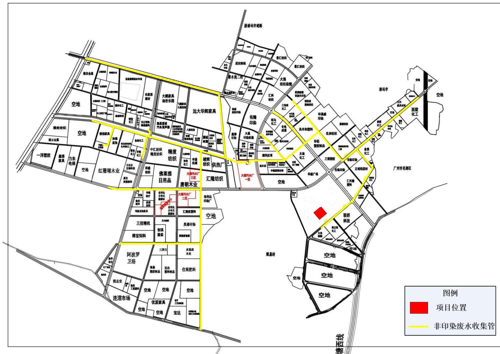
图 5.2-2 大塘污水处理厂非印染废水收集管网图
